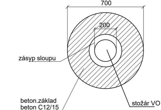
Půdorysný rozměr základu stožáru - prům. 700 mm
